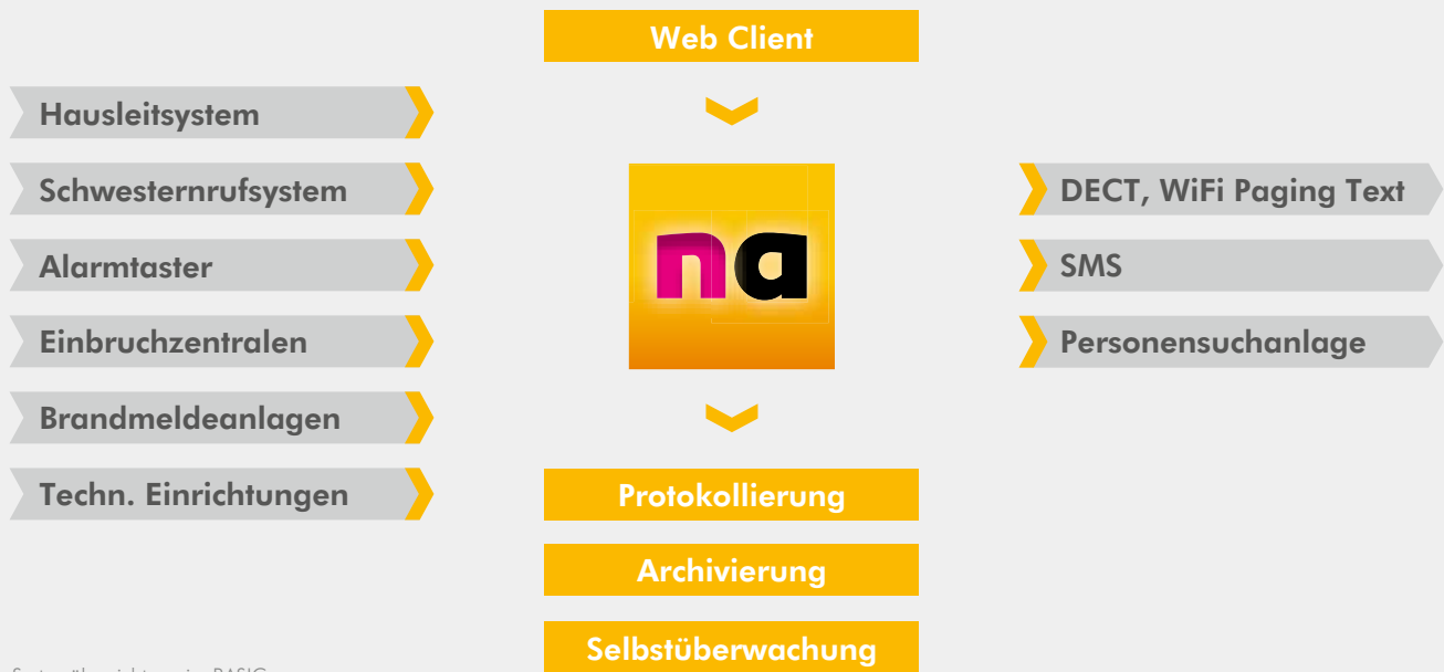
Systemübersicht pagingBASIC
